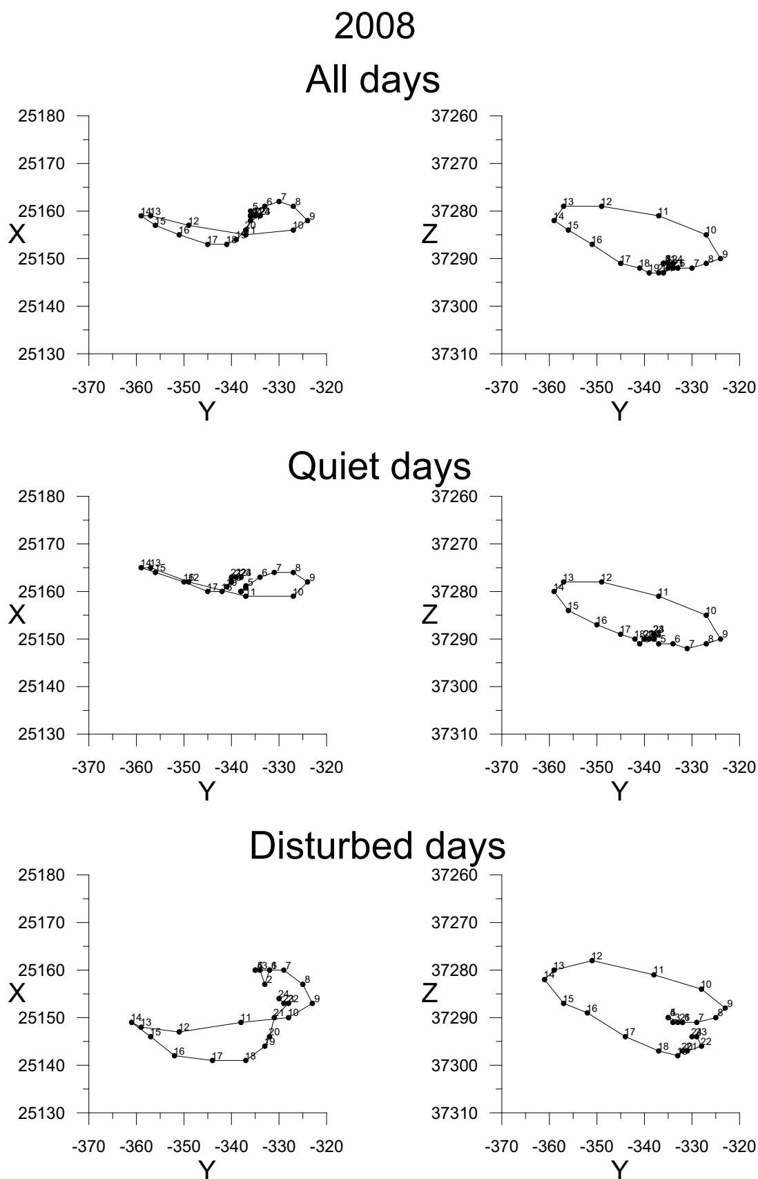
Fig. 4 Hodògrafes de la variació diària en el pla horitzontal i vertical per a tots els dies, els dies de calma i els dies pertorbats. Les unitats són nT. Al costat de cada punt s'indica l'hora corresponent.
